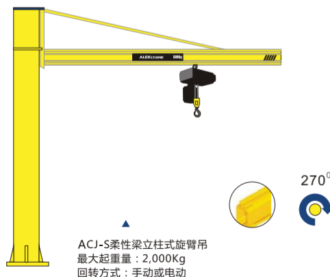
亚历克ACJ-S柔性梁立柱式旋臂吊
