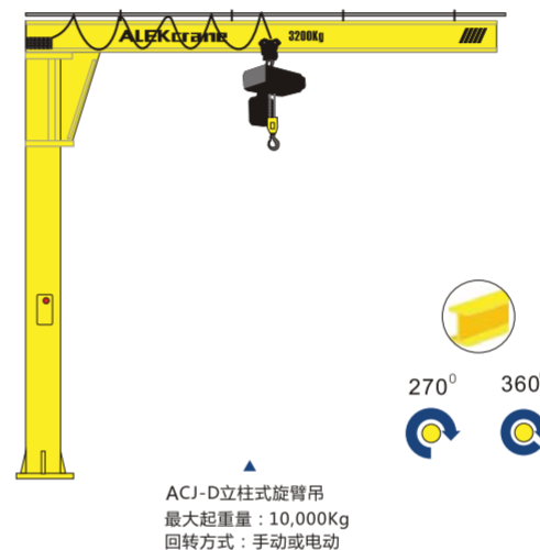
亚历克ACJ-D立柱式旋臂吊
