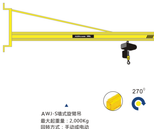
亚历克AWJ-S墙式旋臂吊
