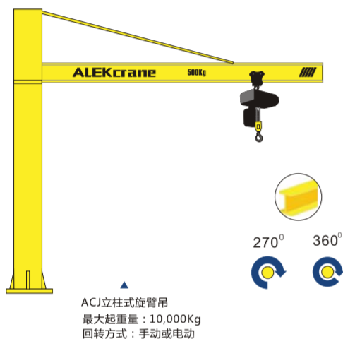
亚历克ACJ-S柔性梁立柱式旋臂吊
